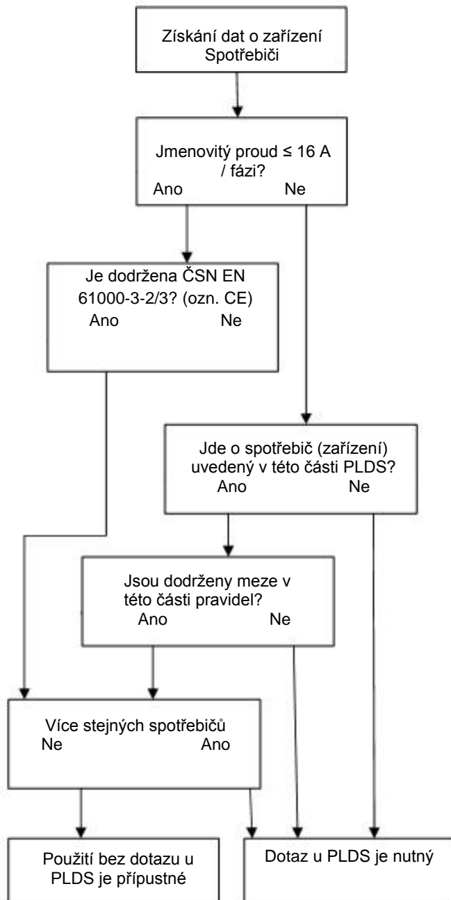
Obr. 1 Schéma po posuzování přístrojů/zařízení se zřetelem na elektromagnetickou kompatibilitu (EMC)
