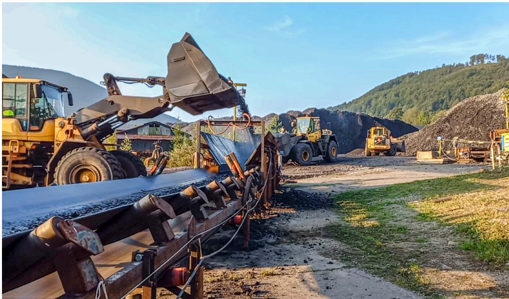
Nakládka zásypového materiálu na dopravníkový pás
