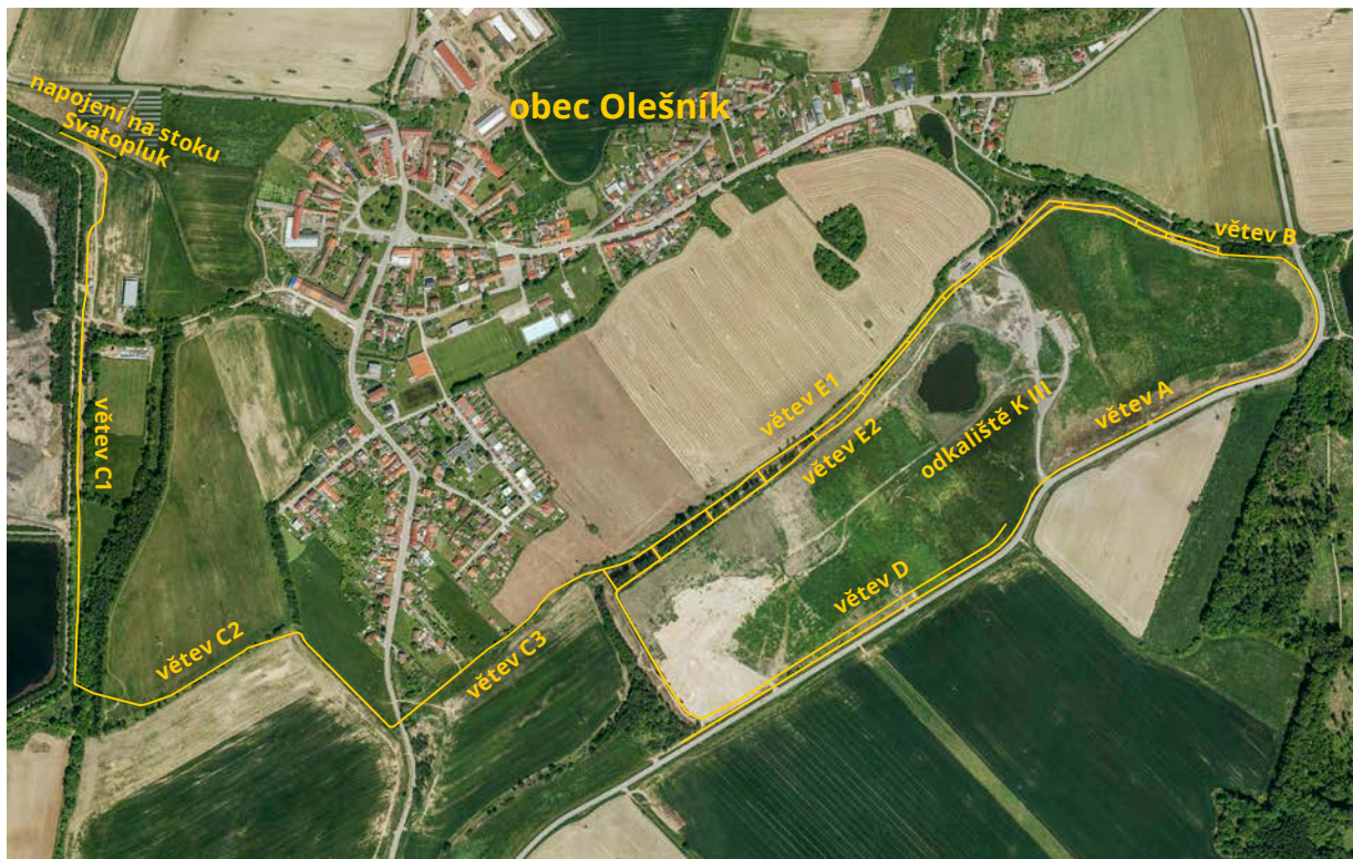
Odvodnění odkaliště K III, přehledná situace stavby
